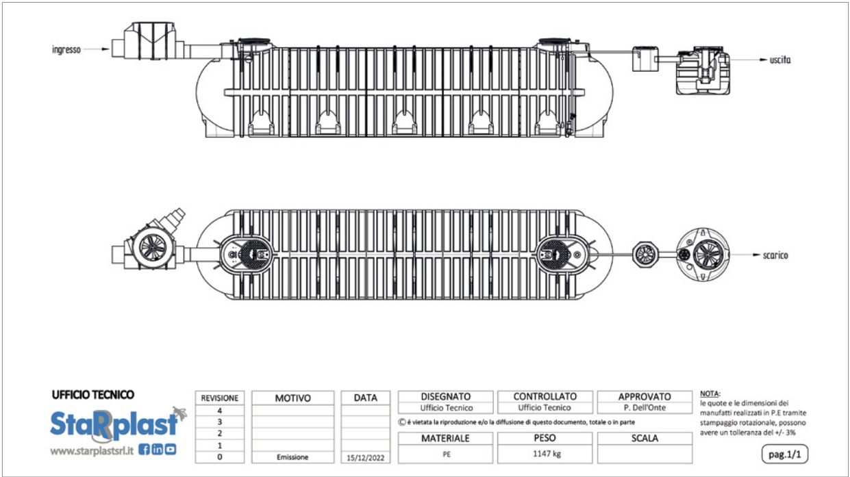
Impianto di prima pioggia in accumulo
