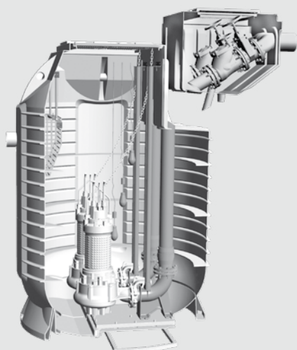
MAXISOL XL
