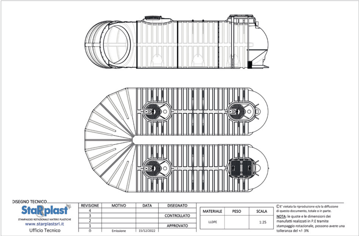
Impianto di laminazione con regolazione di portata in uscita
