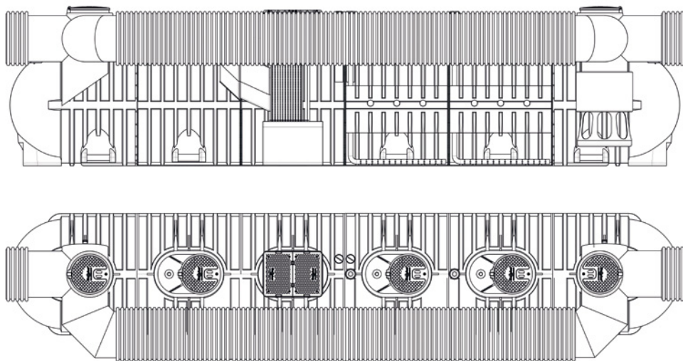
Impianto modulare MB 36.000 con modulo byeplast
