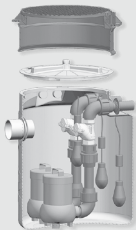
MINISOL DOPPIA POMPA
