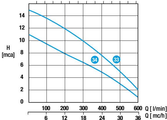
BBC - acque luride
