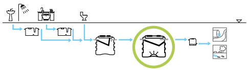
Schema impianto consigliato.
